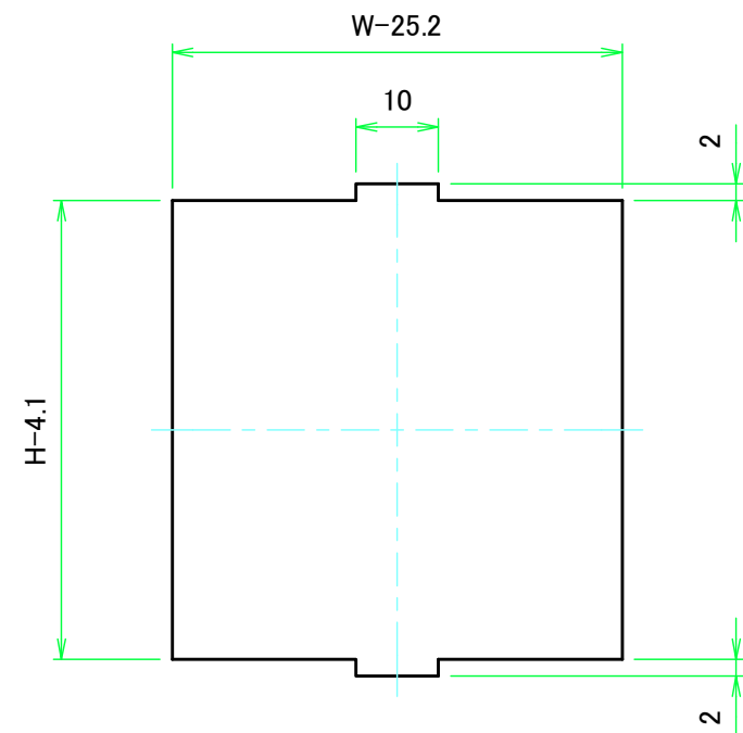
Wパネル1表面 / W Panel 1 Frontside
